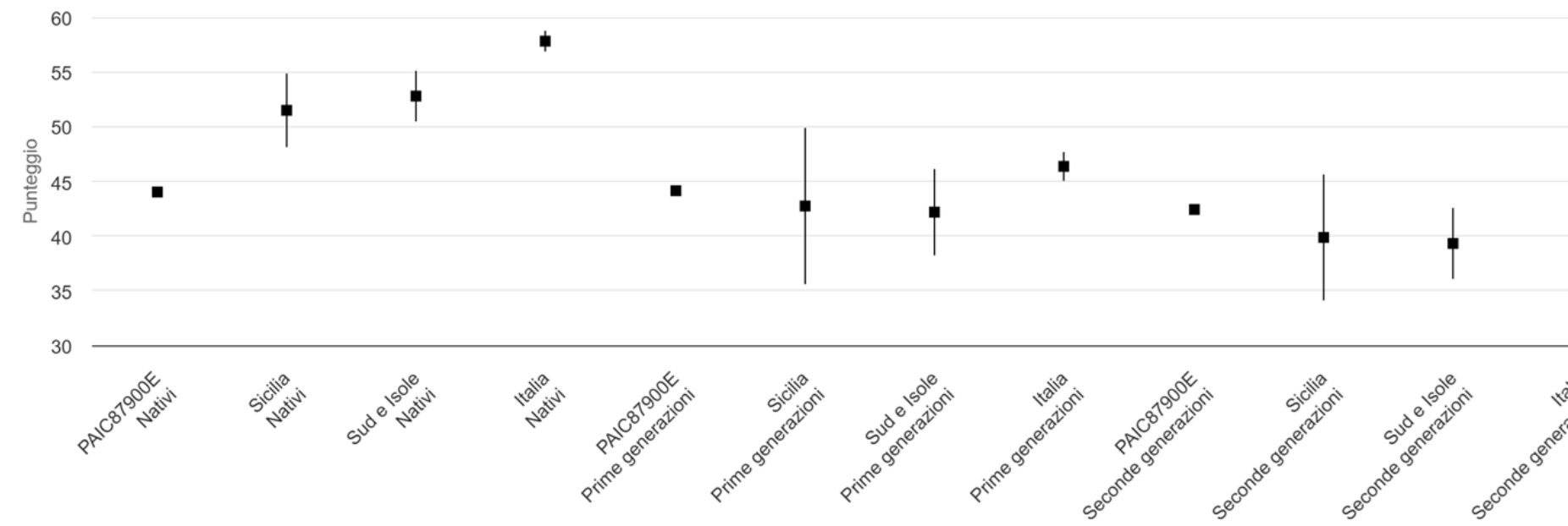
Risultato rispetto all'origine - Matematica classi seconde 2025
